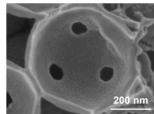
Opale inverse de TiO 2 élaboré par ALD
