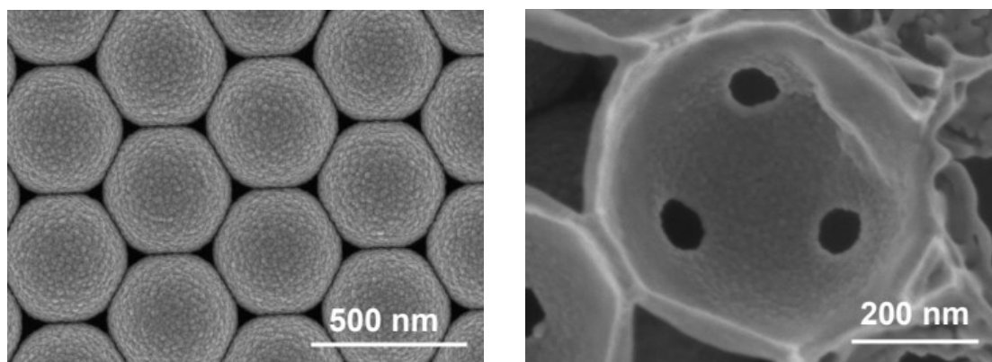
Opale inverse de \text{TiO}_2 élaboré par ALD
